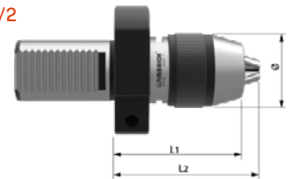
DIN-69893-A [HSK]
